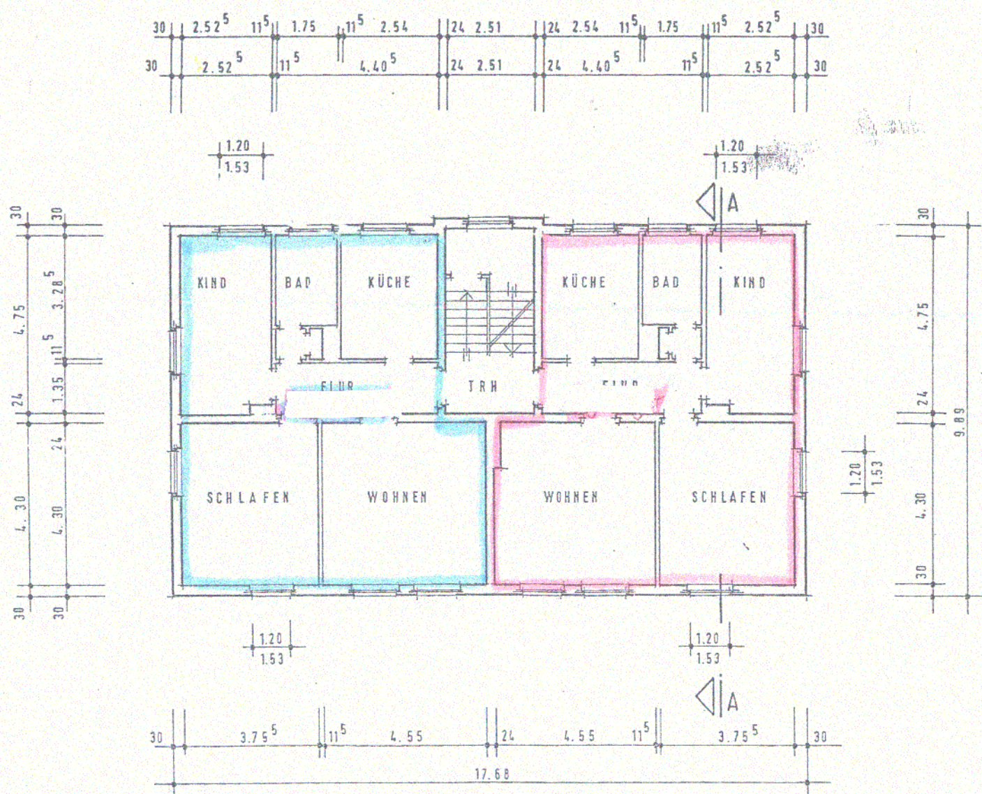
OBERGESCHOSS
