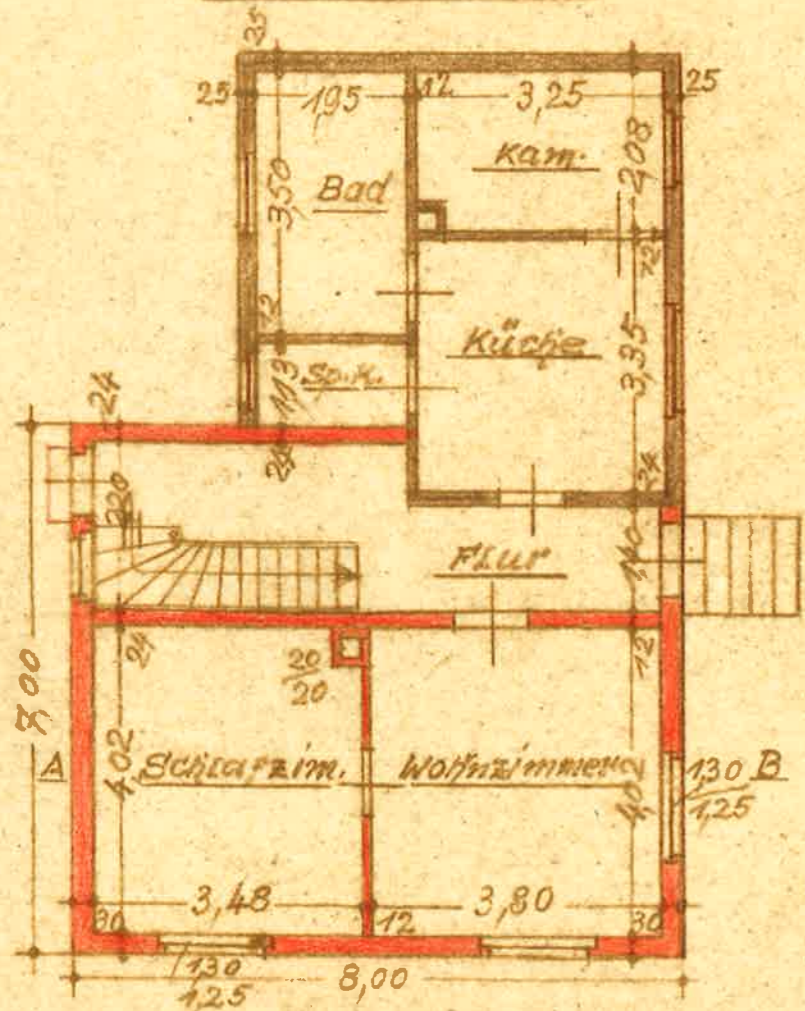
ERDGESCHOSS
