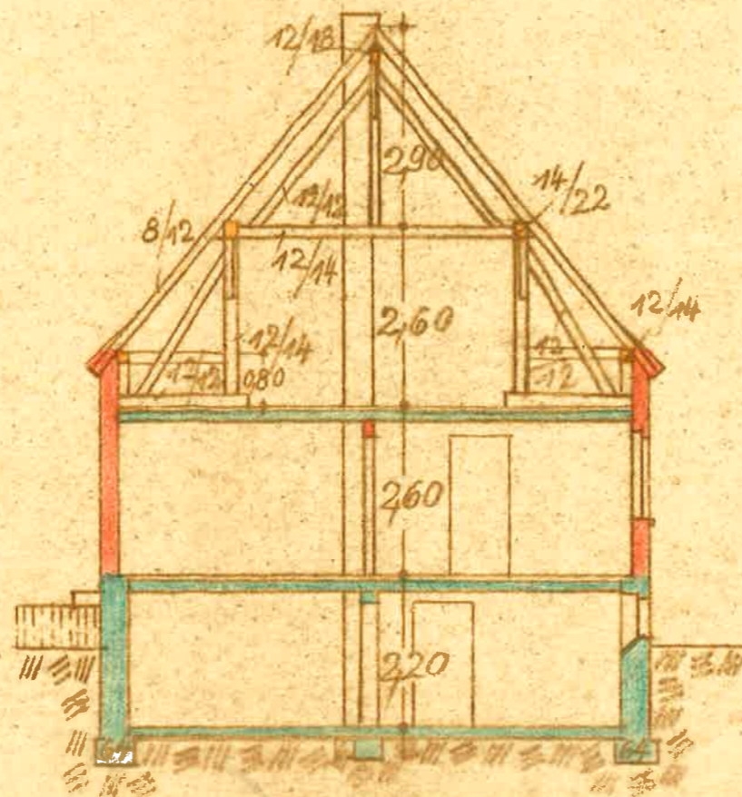
SCHNITT A-B
