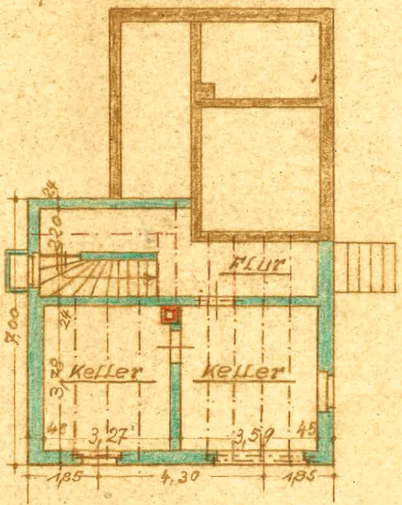
KELLERGESCHOSS
